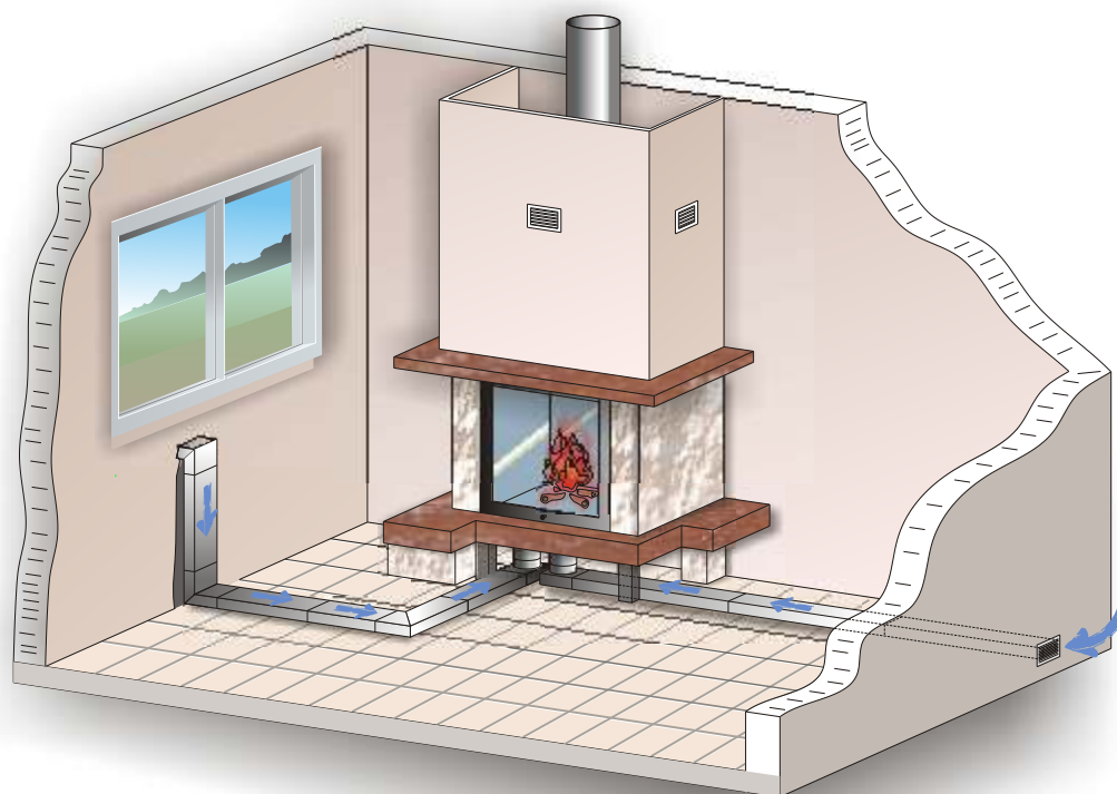
Schema di montaggio
