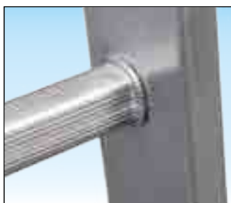
Piolo quadro mm. 30 x 30 anti-scivolo molto robusto con doppia bordatura Unione tra piolo e montante con doppia bordatura, interna ed esterna, per la massima solidità contro urti accidentali ed una lunga durata nel tempo
